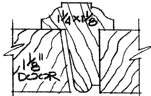
1 1/8" T-ASTRAGAL
